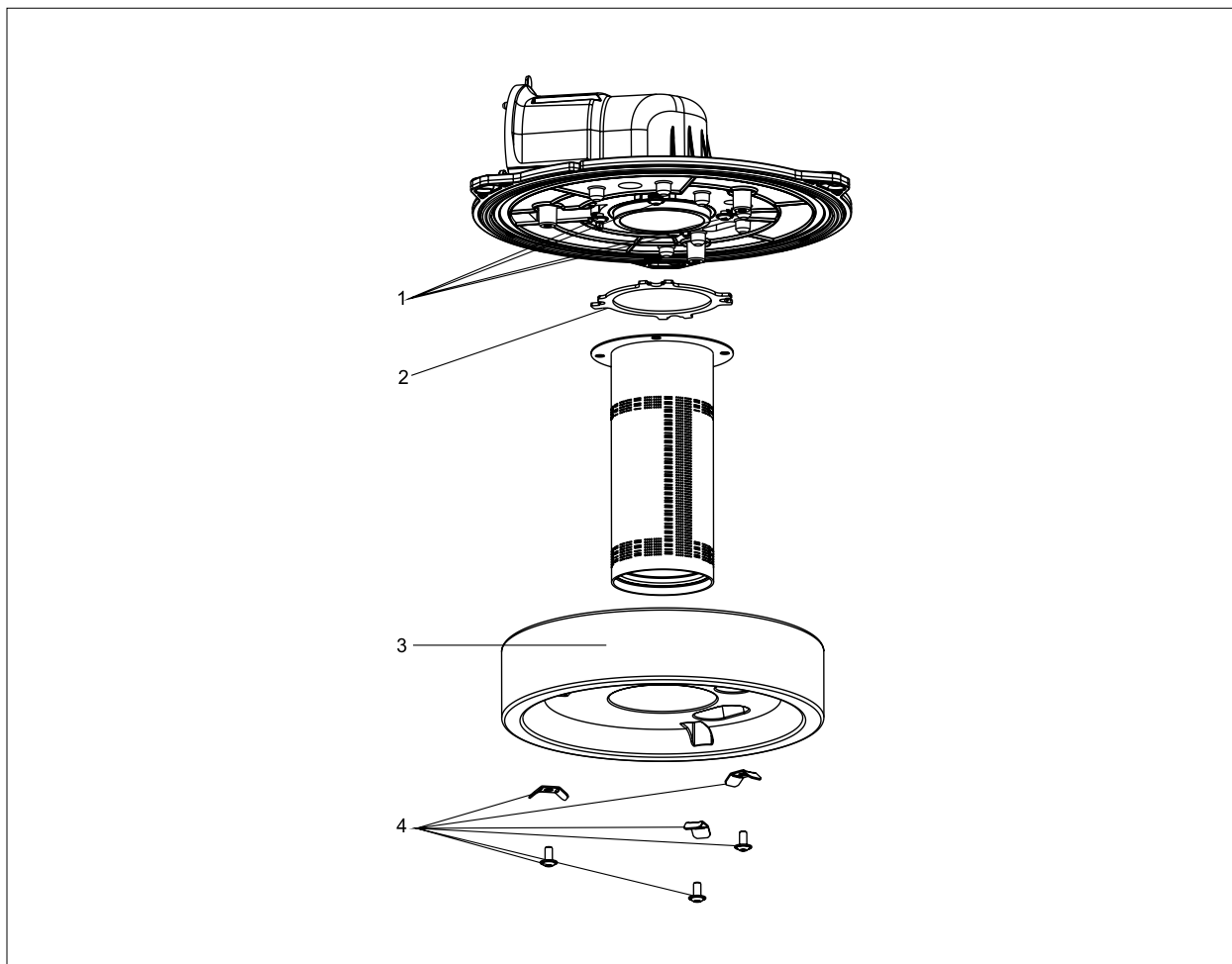
Рис. 6.2 Разборка горелки
