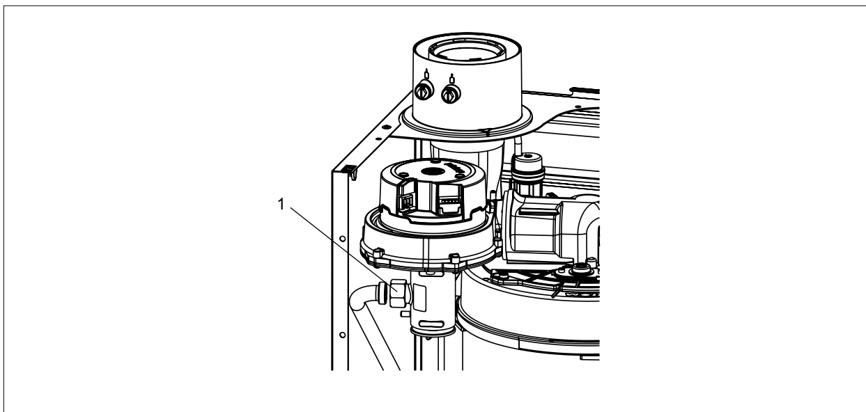
Рис. 5.6 Открывание газовой линии
