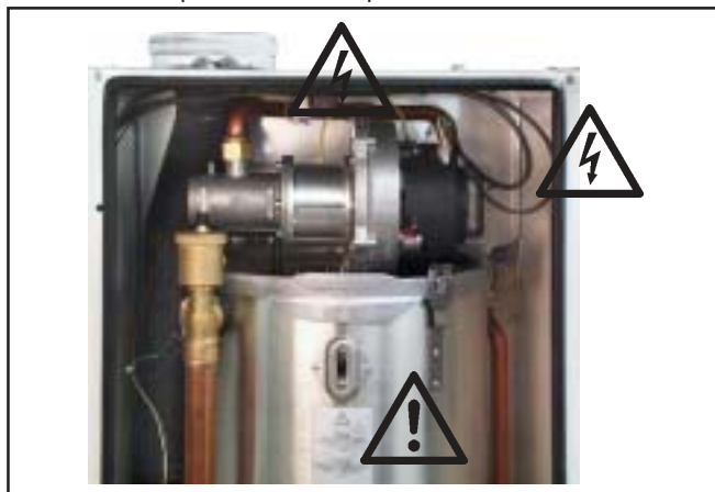
Рис.: Трансформатор поджига, электрод поджига, камера сгорания. Опасность поражения электрическим током, опасность ожога из-за нагретых деталей.
